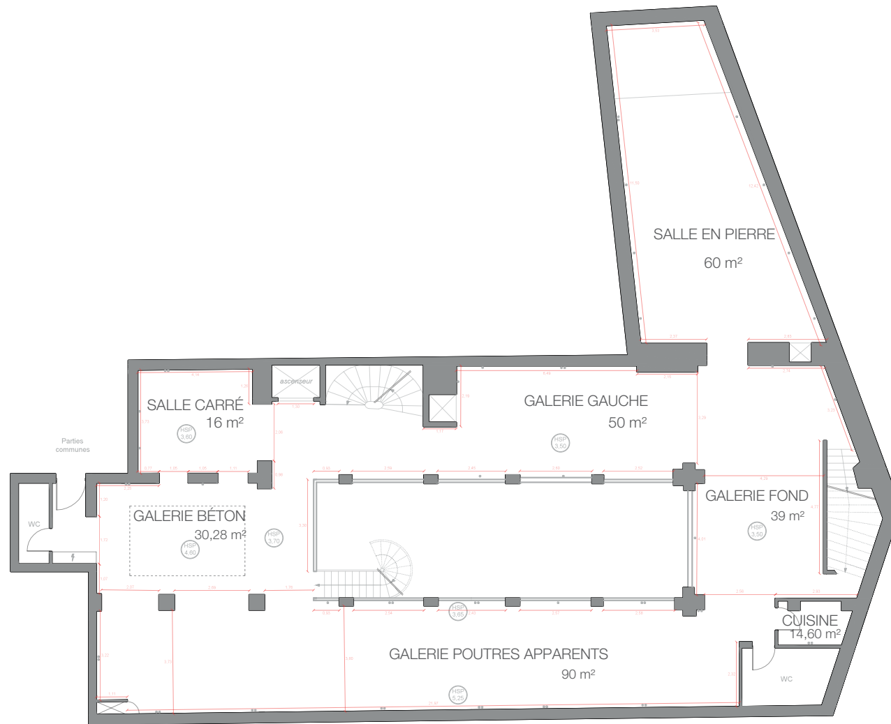
PLAN PREMIER ÉTAGE
